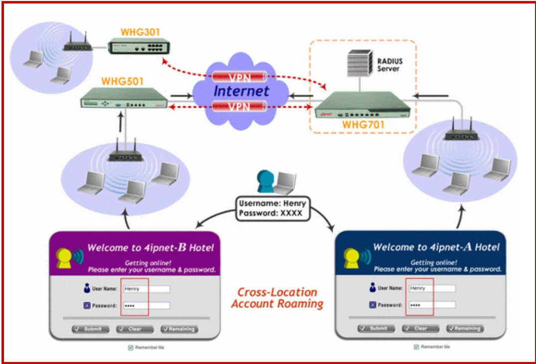
Imagen 2: Roaming de cuentas a través de VPN's a través de dos localizaciones distintas.
